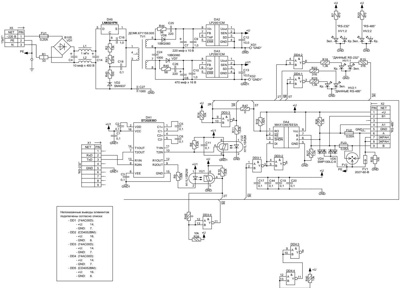
Схема электрическая принципиальная ДСМК.687243.191 ЭЗ [8]
