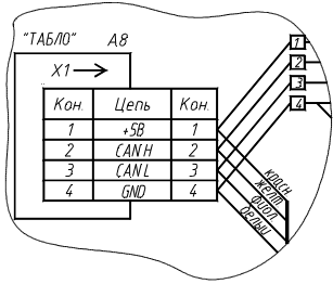
Рис. 2 - Схема подключения устройства индикации Топаз-306БМ2 CAN
