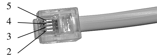
Нумерация контактов вилки 6P4C
