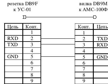
Схема кабеля K2 (из комплекта UC-01)
