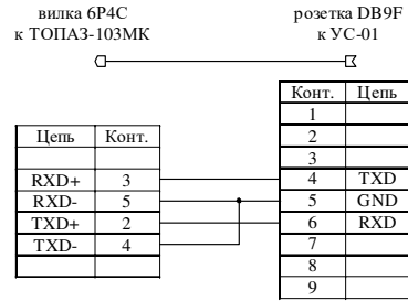
Схема кабеля K1
