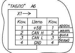
Рис. 2 – устройство индикации "Топаз-306БИ2 CAN". Остальное по рис.1.
